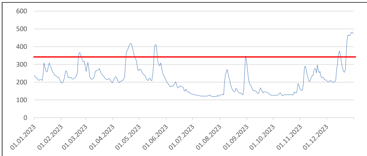
Abbildung 5: Wasserstandentwicklung in der March bei Marchegg in 2023 (in cm; Tagesmittelwerte). Rote Linie: Au wird geflutet (Quelle: Amt der NÖ Landesregierung, abgerufen am 10.1.2024 1 )
